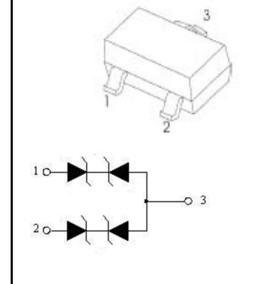
SOT-23
