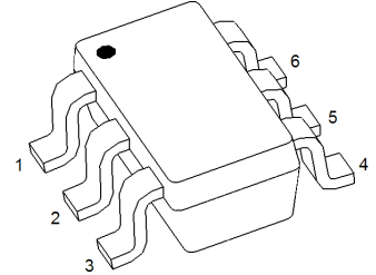
SOT-23-6L
